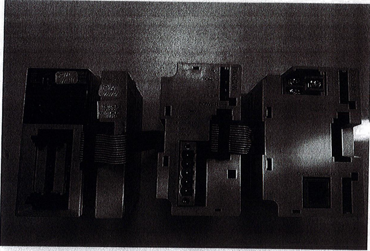
MODÜL 1. ANA PLC MITSUBISHI MELSEC FX 3UC – 16MT/DSS
